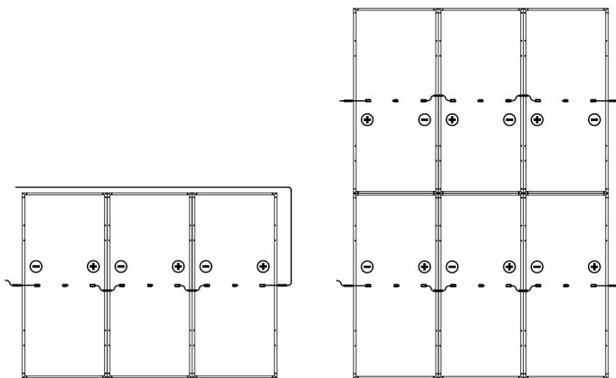
垂直安装
