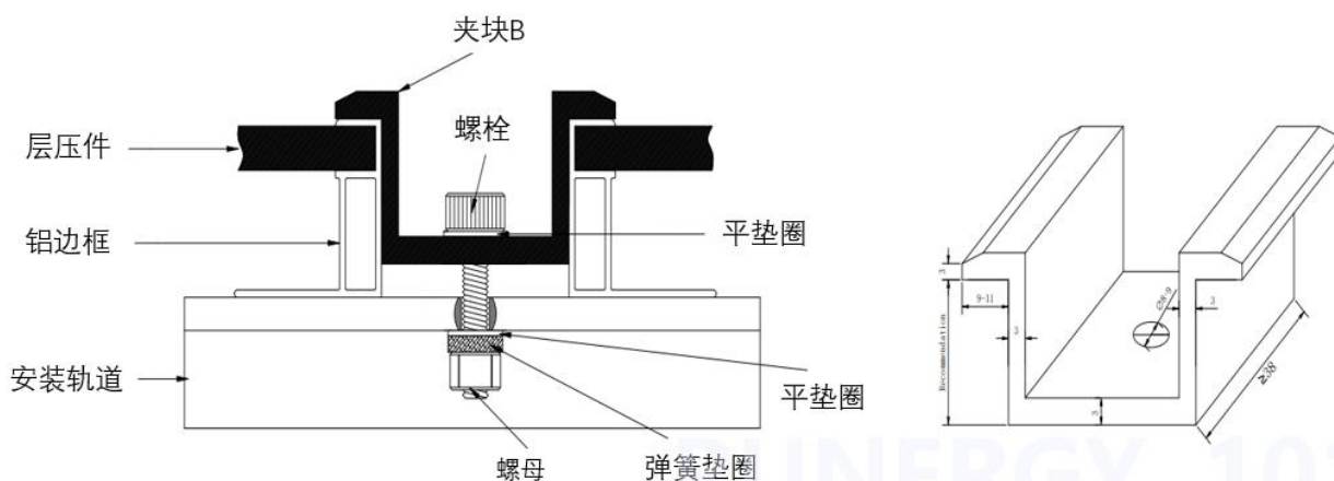
夹块 B
