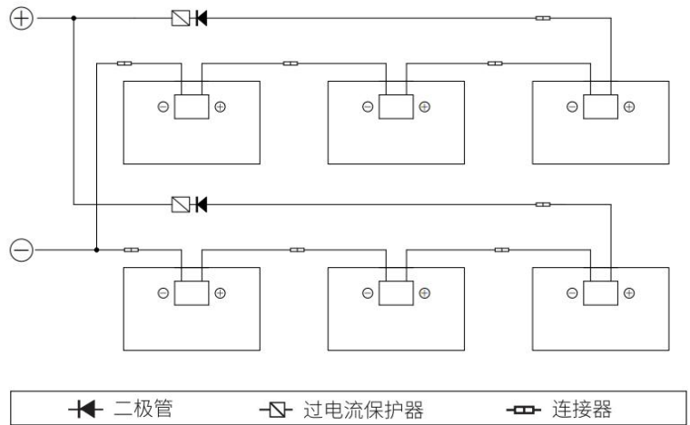
图4：串联和并联接线的电气图
