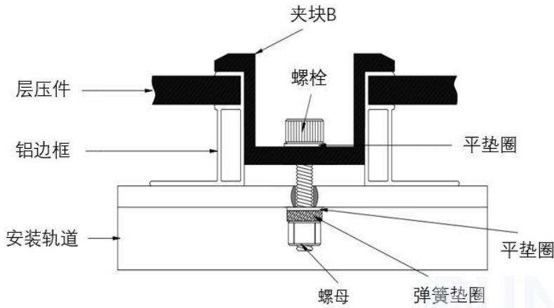
夹块 B
