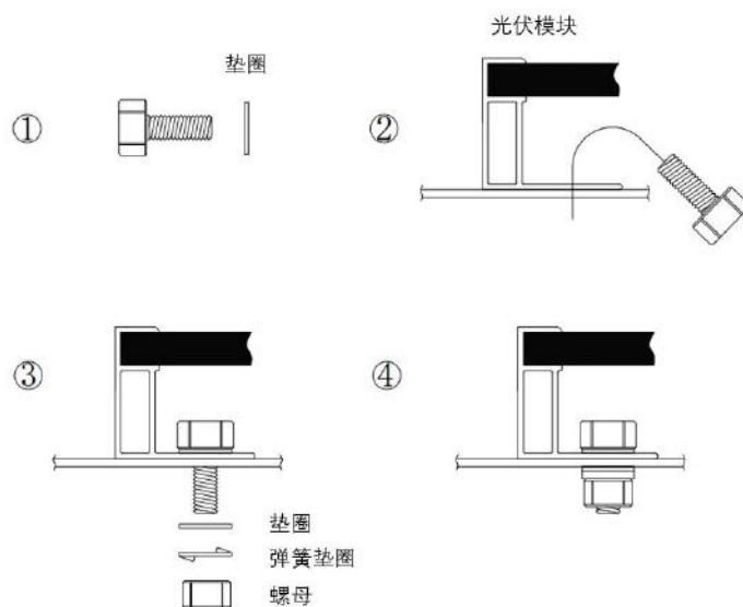
图2：安装细节
