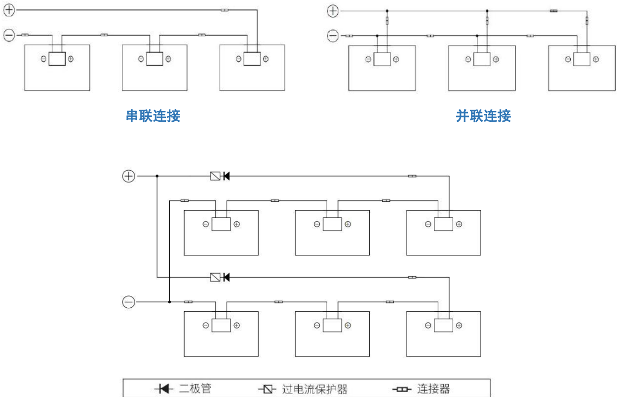
图4：串联和并联接线的电气图
