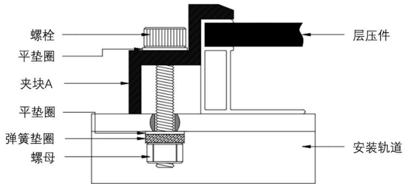
夹块 A
